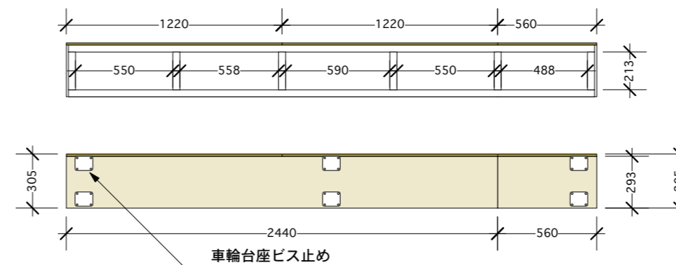
下面図（底側）
