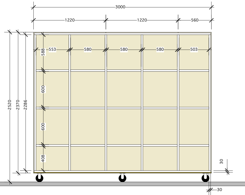
背面図（バックヤード側）
