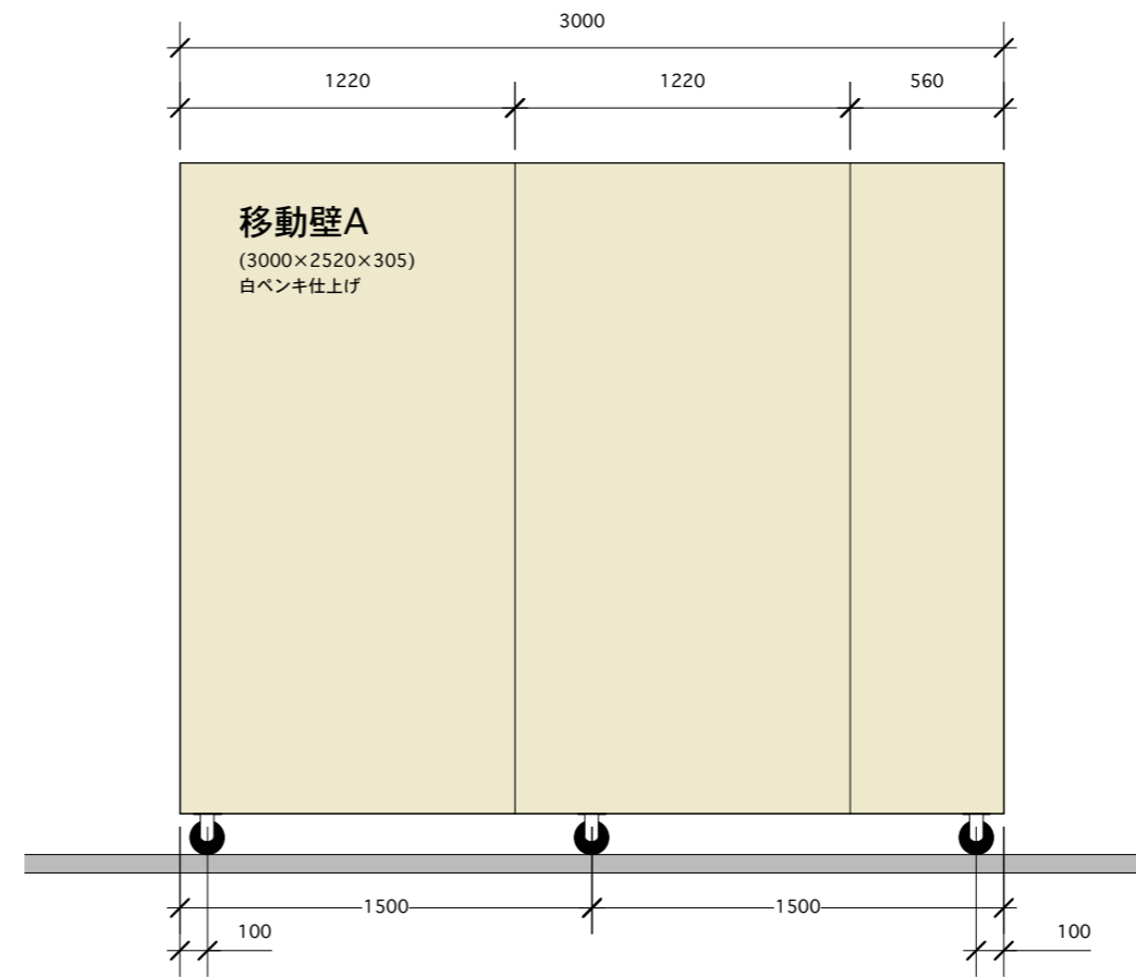
正面図
