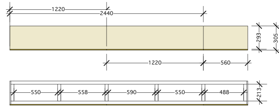
平面図（天井側）
