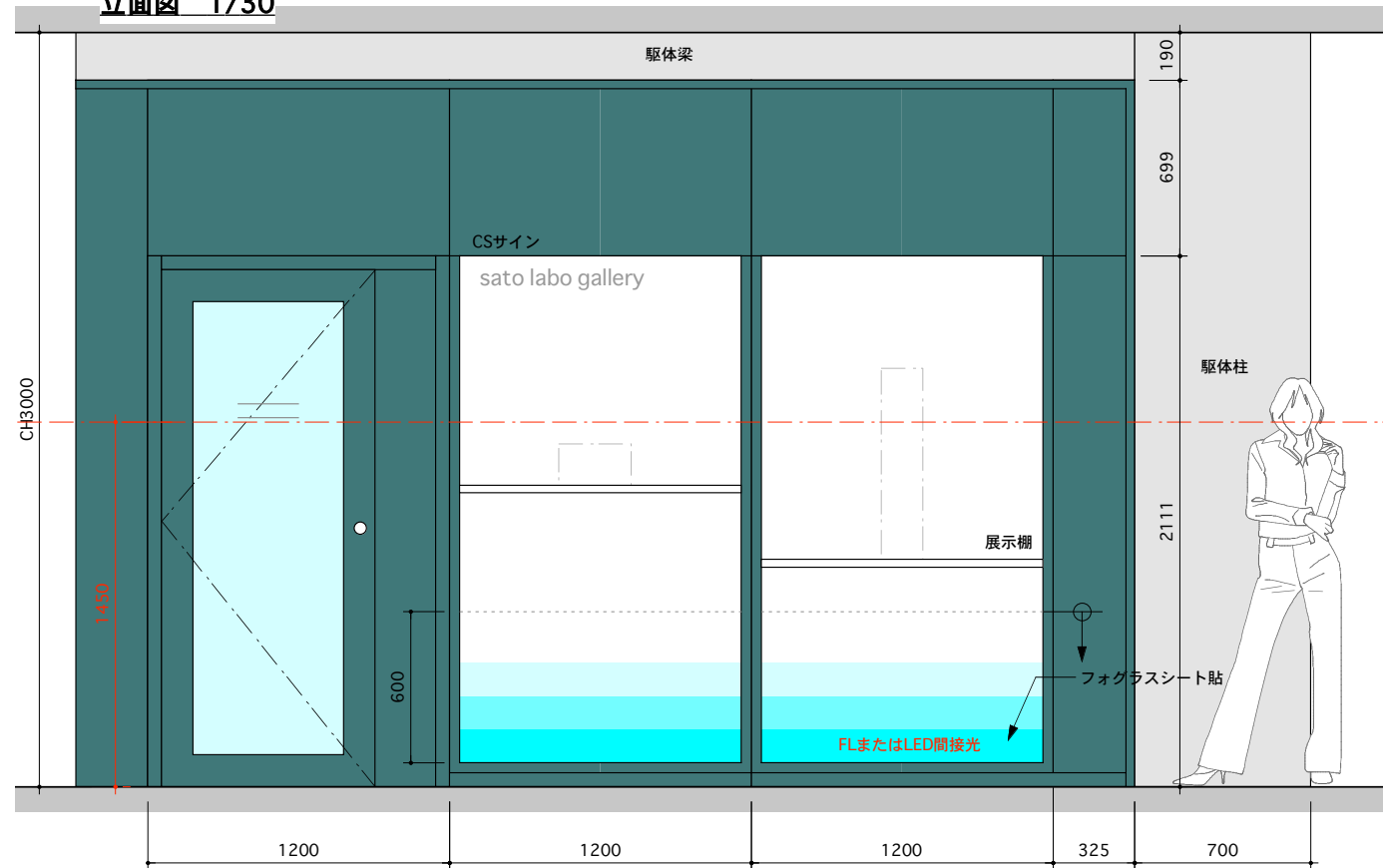
立面図 1/30
