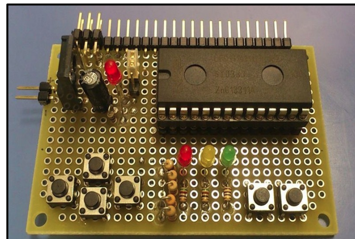
③ mbedを使った マイコンボード 「がちゃコンボード」
