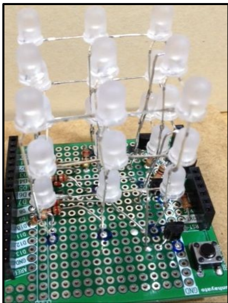
① Arduinoを使った LEDキューブ
